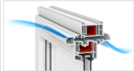
Druckgesteuertes Zuluftelement Aereco AMO
