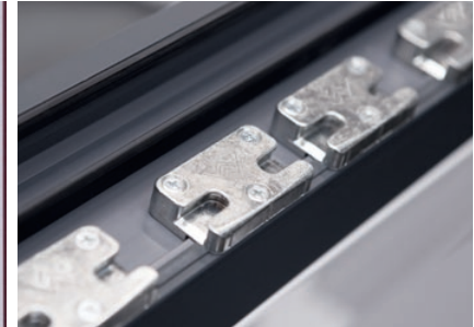
Einbruchsicherer Haken im Dreh-Kipp-Flügel (RU)
