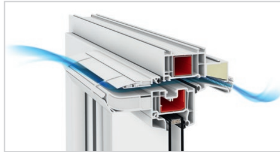
Hygrostatisch gesteuertes Zuluftelement EXR 409
