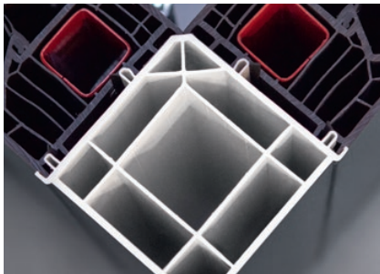
Verbinder
